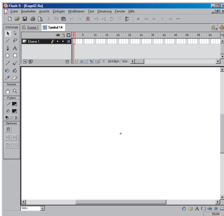
Der Symbolbearbeitungsmodus
