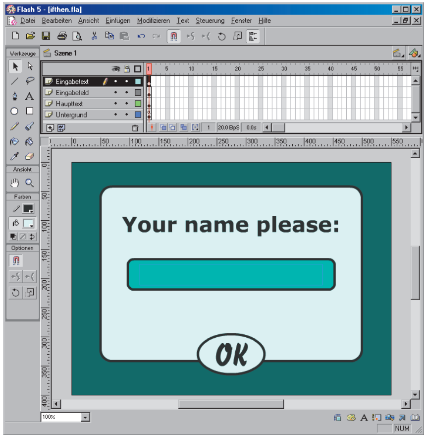
Die Vorlage
