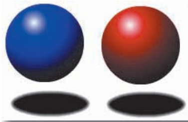
Das Endergebnis
