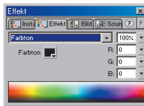
Das Effekt-Bedienfeld
