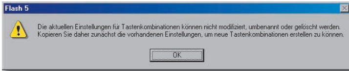
Gesperrte Tastenkürzelzusammenstellungen
