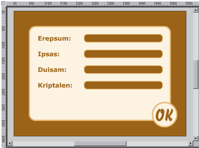
Das Zwischenstadium
